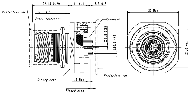
TV07 UCOM CI * -11 S F459
