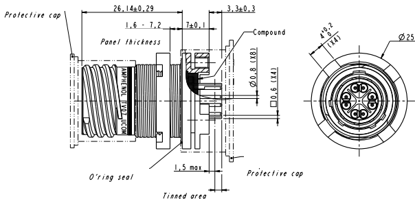
TV07 UCOM CI * -11 S F059
